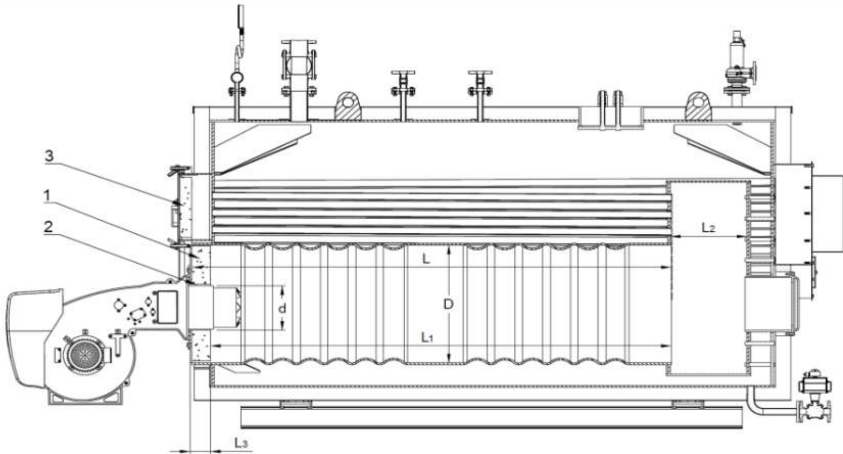
Присоединительные размеры.
